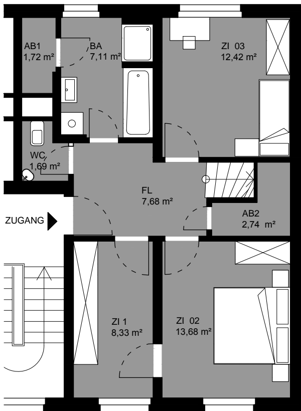
4. Obergeschoss
